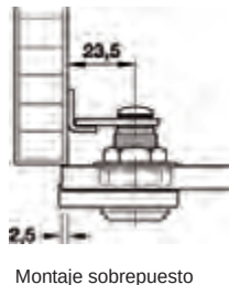
Montaje sobrepuesto
