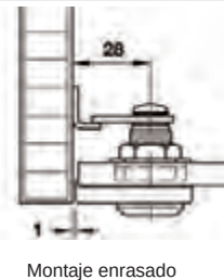
Montaje enrasado
